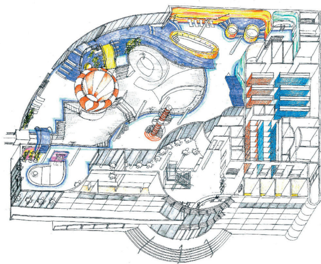
„Pracovní skica barevné axonometrie interiérů Aquaparku Olomouc“ Autoři Ing. arch. Jan Vrána, HÉTA – architektonický ateliér a Stavoprojekt Olomouc a. s.
